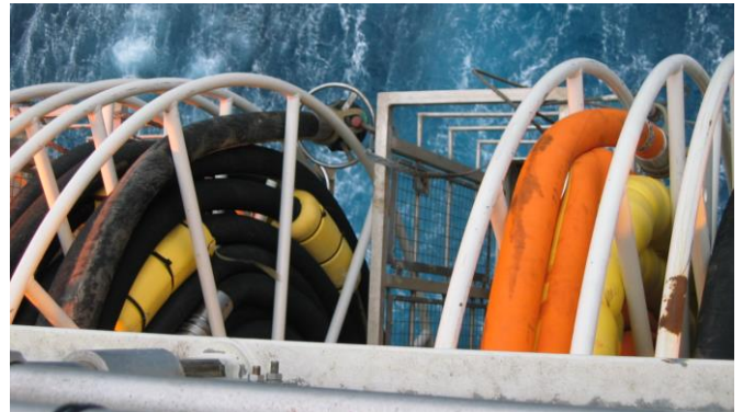
Figur 7.5: Bunkringsslange for drikkevann. Slangen har lys farge for å redusere oppvarming. Begge slangene på bildet har flytelementer for å hindre at de skal komme inn i forsyningsbåtens propeller (Foto: Eyvind Andersen)
