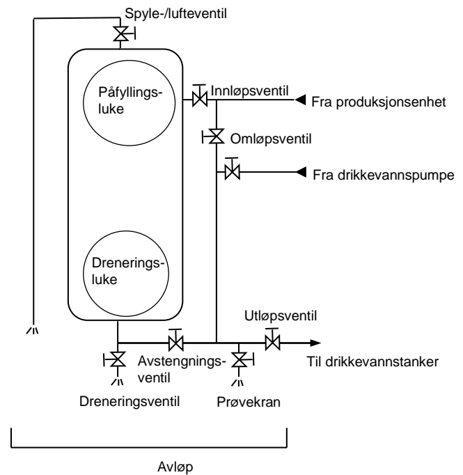
Figur 8.1: Filteret må bygges slik at det er lett å komme til ved rengjøring, utskifting av masse og annet vedlikehold (Ill.: Karin Melsom)
