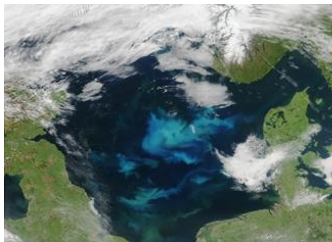
Figur 6.1: Intense planktonoppblomstringer i sommerhalvåret, her observert i Nordsjøen fra NASAs jordobservatorium, kan av og til føre til lukt- og smaksproblemer på innretninger som produserer drikkevann (Foto: NASA/Jesse Allen)
