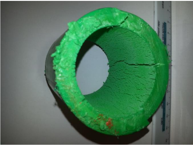
Figur 9.20: Varmtvannsrør som har blitt ødelagt som følge av manglende ekspansjonskar og en kombinasjon av høyt trykk og høy temperatur i varmtvannsnettet. (Foto: Johan Ljungqvist)
