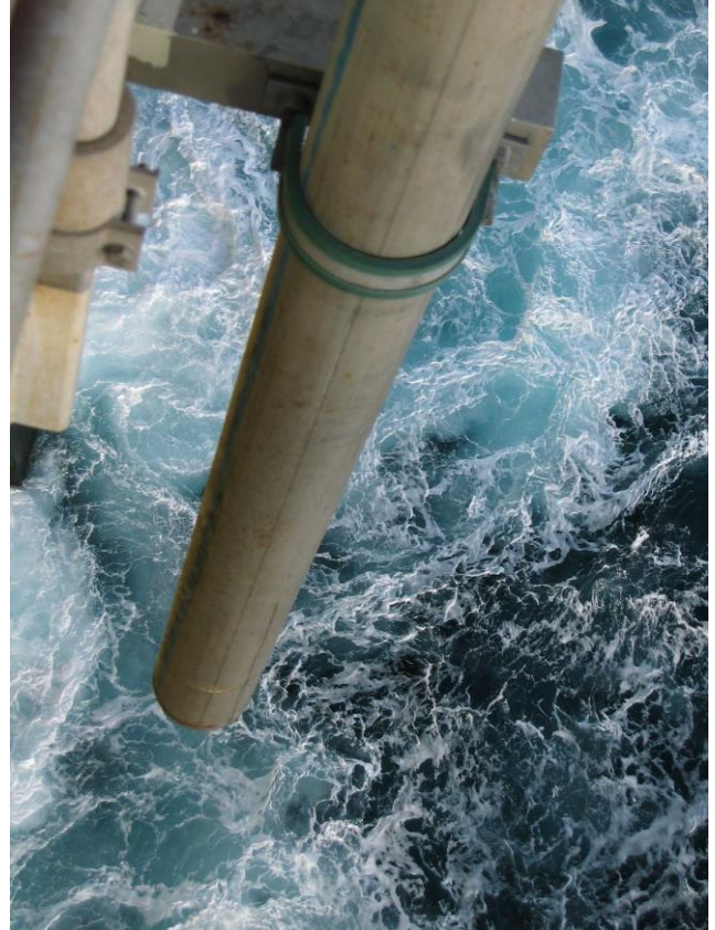
Figur 7.9: Når spylørøret er av samme dimensjon som bunkringsslangen får man spylt med fullt trykk (Foto: Eyvind Andersen)
