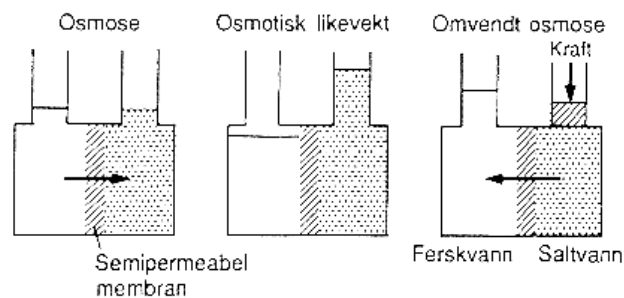
Figur 6.6: Figuren viser hvordan prinsippet for osmose og omvendt osmose fungerer (Ill. hentet fra B3/NIVAs tegnekontor)
