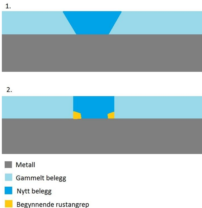
Figur 9.9: Tverrsnitt 1 viser korrekt flekkmaling, hvor kant mellom nytt og gammelt belegg er pusset ned. Tverrsnitt 2 illustrerer begynnende korrosjon som følge av manglende pussing, og hvor «rette kanter» gjør at man ved påføring av belegg ikke kommer til alle steder inn mot stålet selv om man bruker pensel (Ill. Eyvind Andersen)
