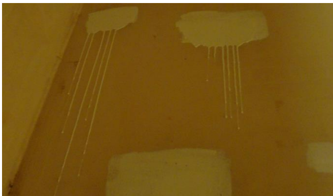
Figur 9.10: Feil utført flekkmaling. Man har brukt rull i stedet for rund pensel og belegget er «klist utover» i tykke lag (Foto: Bjørn Løfsgaard)
