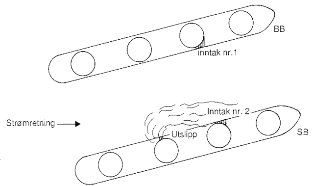
Figur 6.3: Sjøvannsinntak må ikke plasseres nedstrøms utslipp med den strømningsretning som er vanlig i området. Inntak bør ikke ligge på samme side som utslipp, og burde her vært flyttet til utsiden av pongtongene (Ill.: NIVAs tegnekontor)
